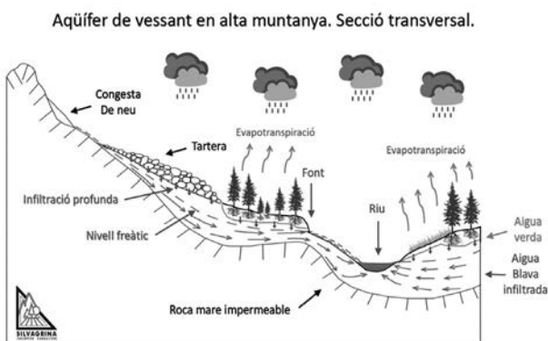
Figura 2. Esquema simplificat del funcionament d'un aqüífer de vessant en alta muntanya, per a la producció d'aigua blava infiltrada, que és la que estima el model de l'hidrogràfic sintètic de recés proposat
